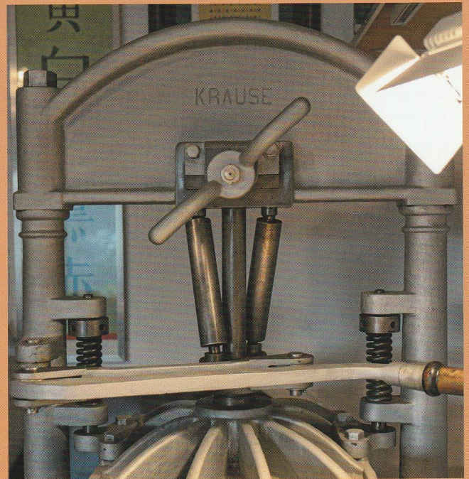
Josua Reicherts Kniehebelpresse in seiner Werkstatt, Foto © Laura Reichert
